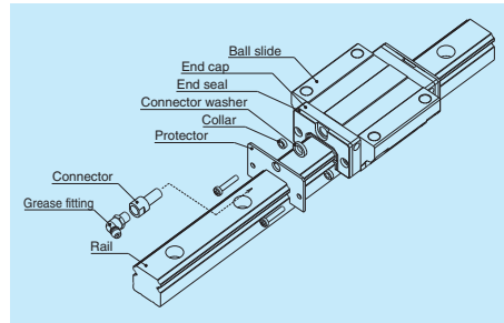
Fig. 15 Protector
